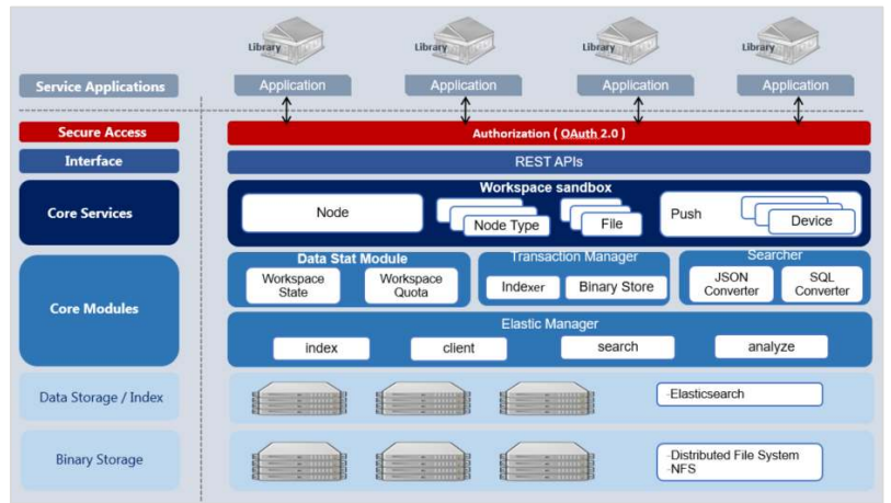
[S/W 시스템 구성도]
